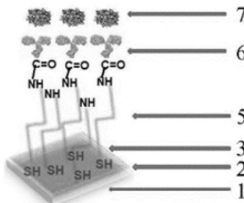
Rys. 1. Schemat biosensora do oznaczania interleukiny 6 (IL6)
